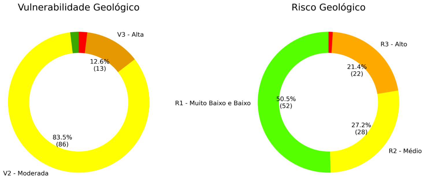
Figura 5.1-1. Porcentagem e valores absolutos de risco e vulnerabilidade a processos geológicos do município de Caçapava.
