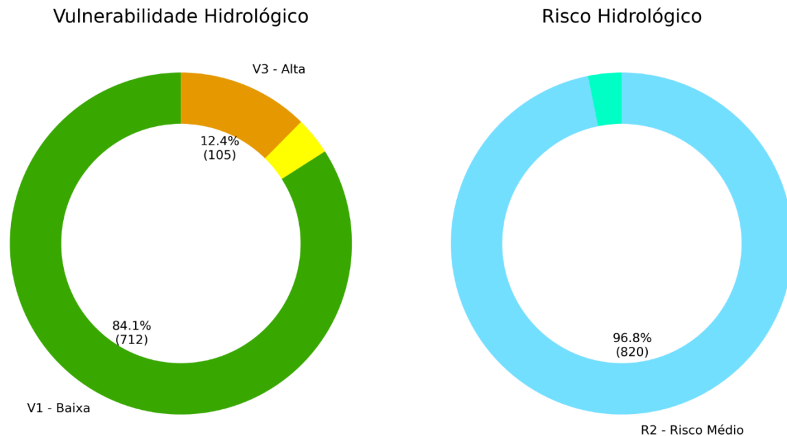
Figura 6.1-1. Porcentagem e valores absolutos de risco e vulnerabilidade a processos hidrológicos do município de Caçapava.
