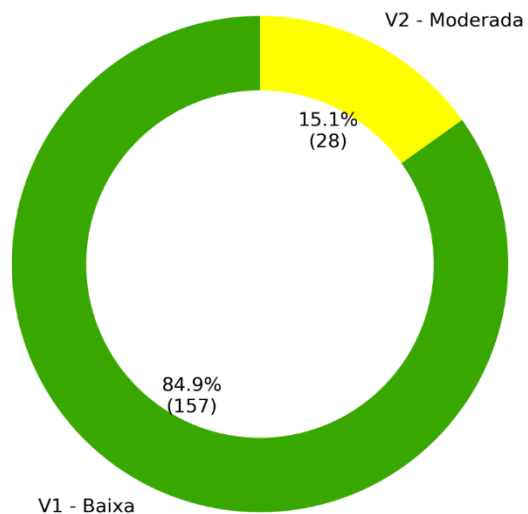
Figura 6.1-1. Porcentagem e valores absolutos de risco e vulnerabilidade a processos hidrológicos do município de Canas.
