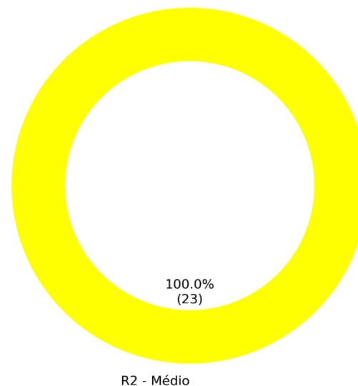
Figura 5.1-1. Porcentagem e valores absolutos de risco e vulnerabilidade a processos geológicos do município de Canas.
