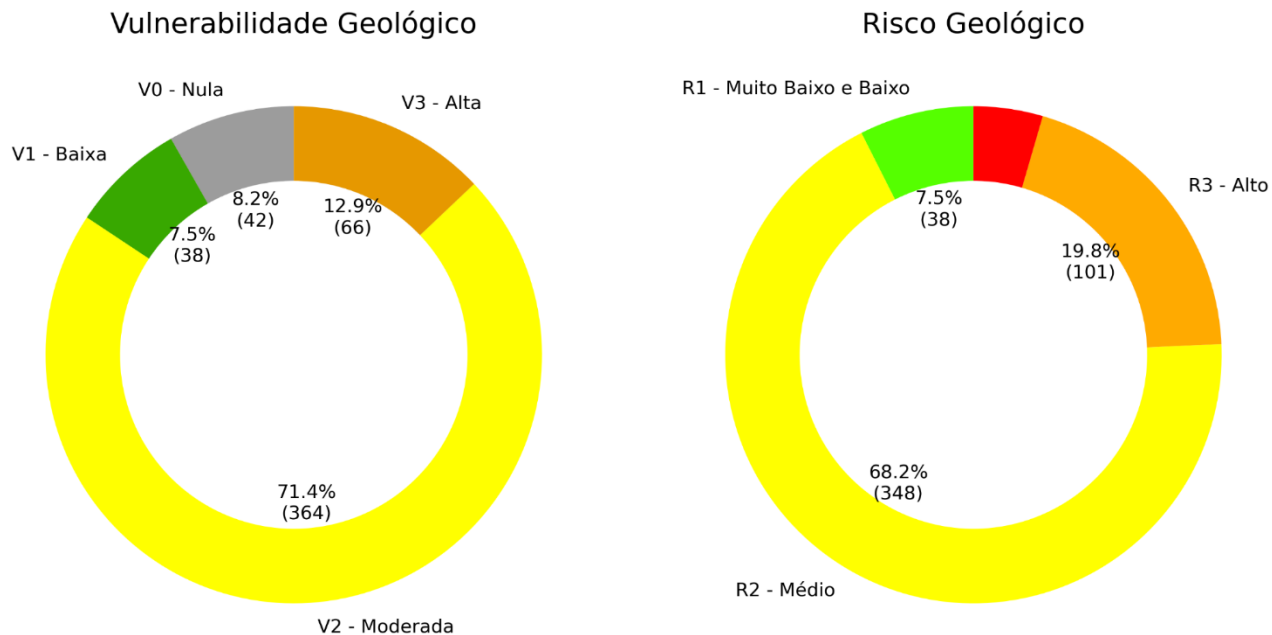
Figura 5.1-1. Porcentagem e valores absolutos de risco e vulnerabilidade a processos geológicos do município de Guararema.
