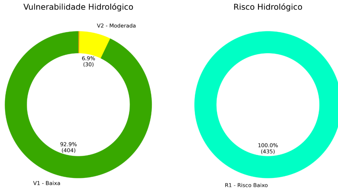
Figura 6.1-1. Porcentagem e valores absolutos de risco e vulnerabilidade a processos hidrológicos do município de Guararema.
