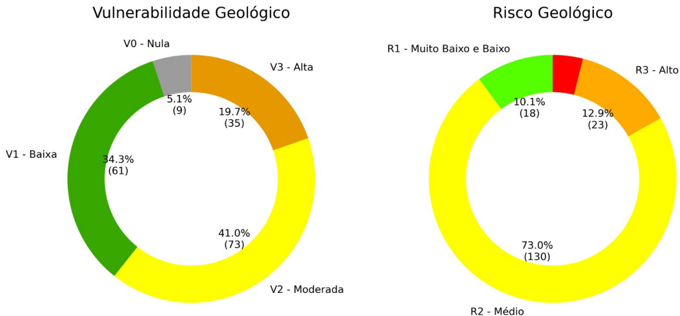
Figura 5.1-1. Porcentagem e valores absolutos de risco e vulnerabilidade a processos geológicos do município de Monteiro Lobato.
