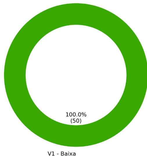
Figura 6.1-1. Porcentagem e valores absolutos de risco e vulnerabilidade a processos hidrológicos do município Natividade da Serra.
