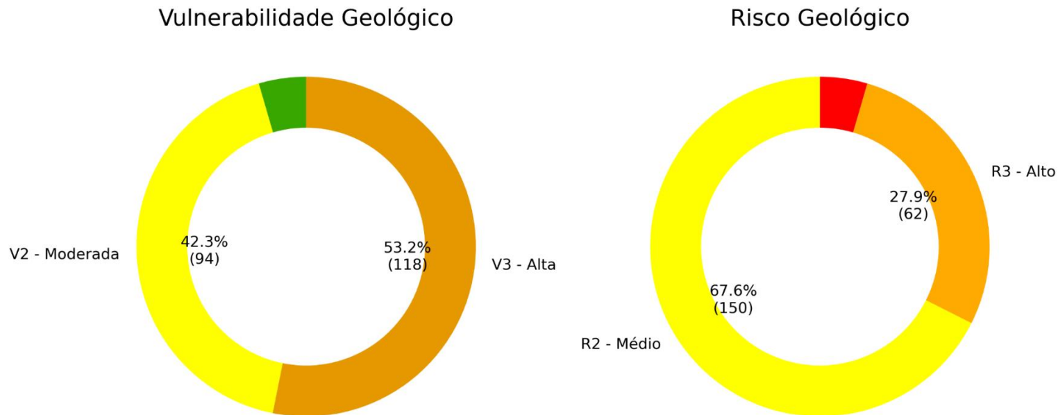
Figura 5.1-1. Porcentagem e valores absolutos de risco e vulnerabilidade a processos geológicos do município de Natividade da Serra.
