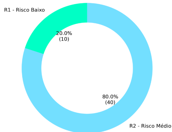
Figura 6.1-1. Porcentagem e valores absolutos de risco e vulnerabilidade a processos hidrológicos do município Natividade da Serra.
