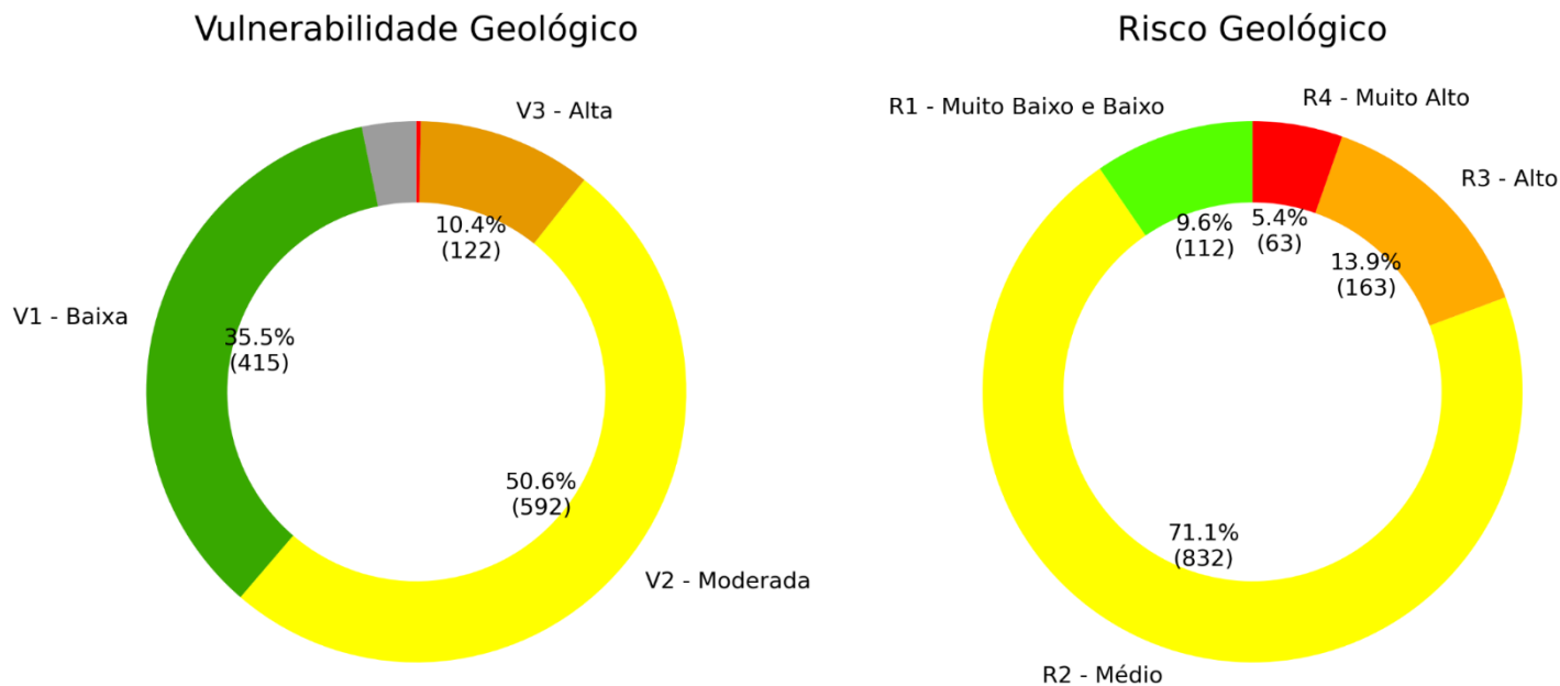
Figura 5.1-1. Porcentagem e valores absolutos de risco e vulnerabilidade a processos geológicos do município Paraibuna.
