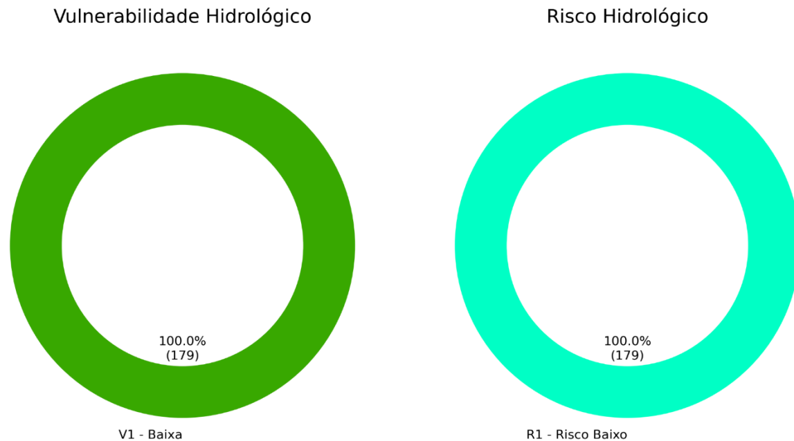
Figura 6.1-1. Porcentagem e valores absolutos de risco e vulnerabilidade a processos hidrológicos do município de Santa Isabel.
