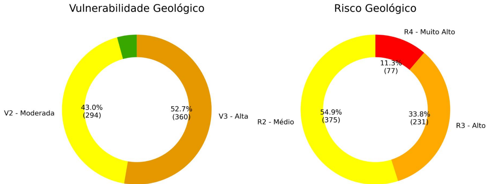
Figura 5.1-1. Porcentagem e valores absolutos de risco e vulnerabilidade a processos geológicos do município de Santa Isabel.
